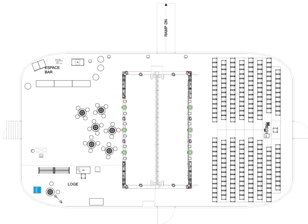
Plan aérien du chapiteau en composition gradins
